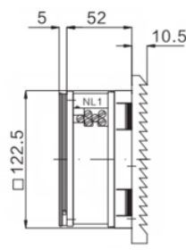
侧视图(入口) Side View(Inlet)
